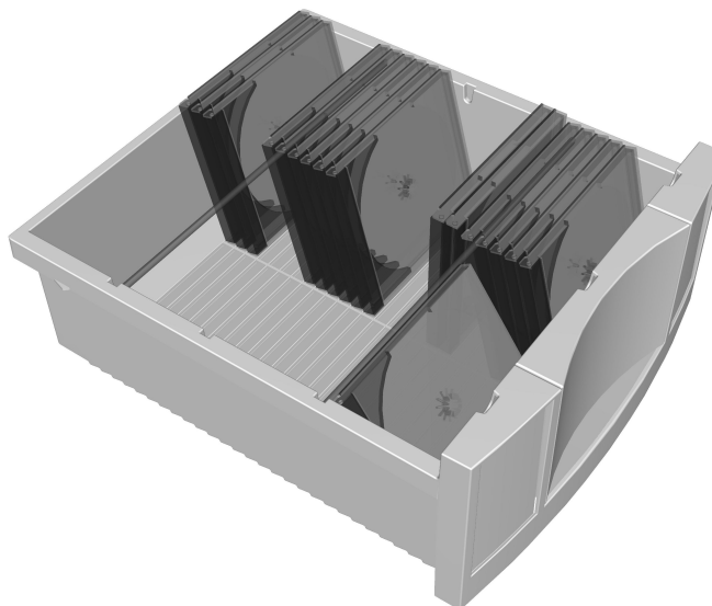
Vue intérieure du tiroir H.150mm pour CD
